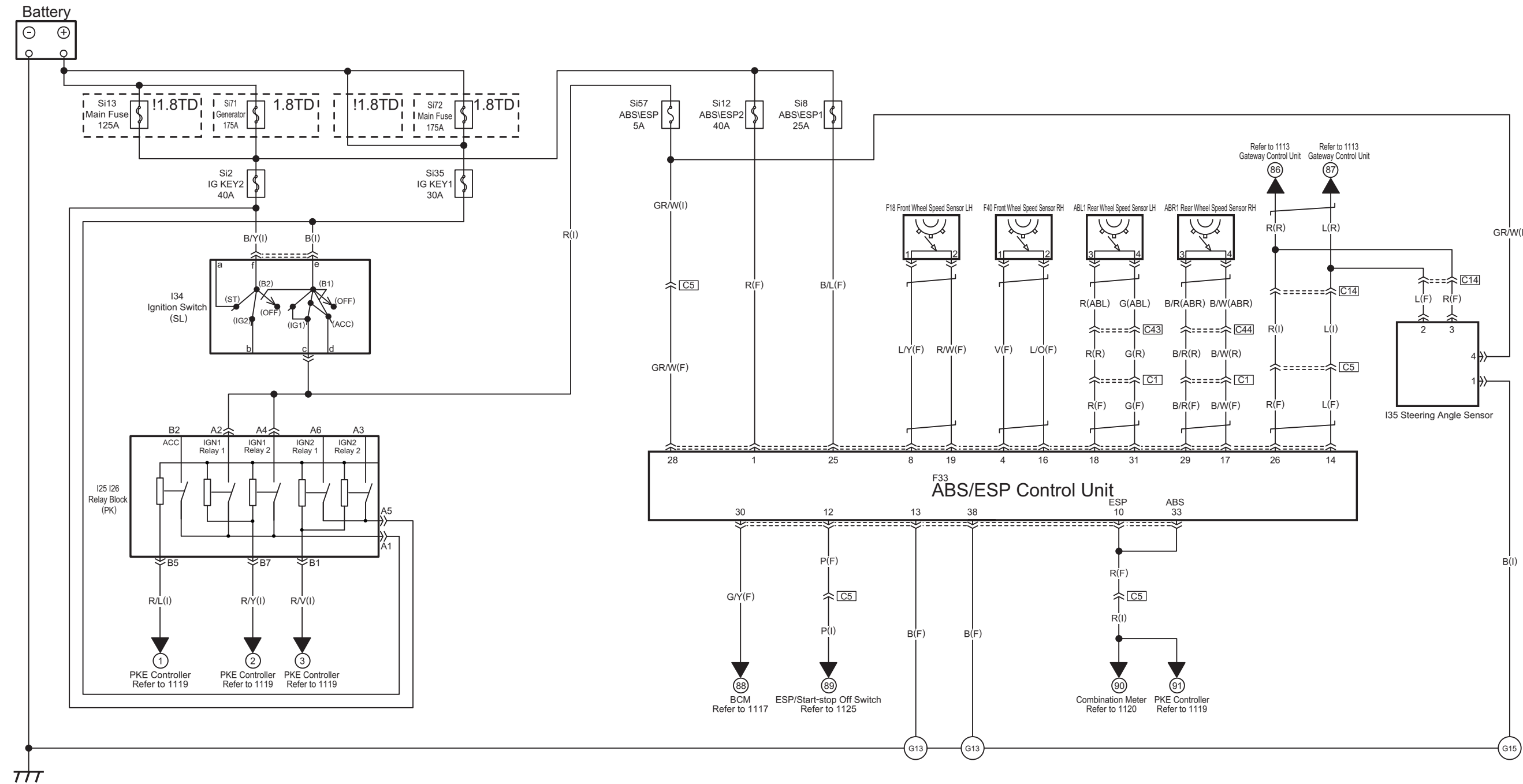
F33 ABS/ESP Control Unit
